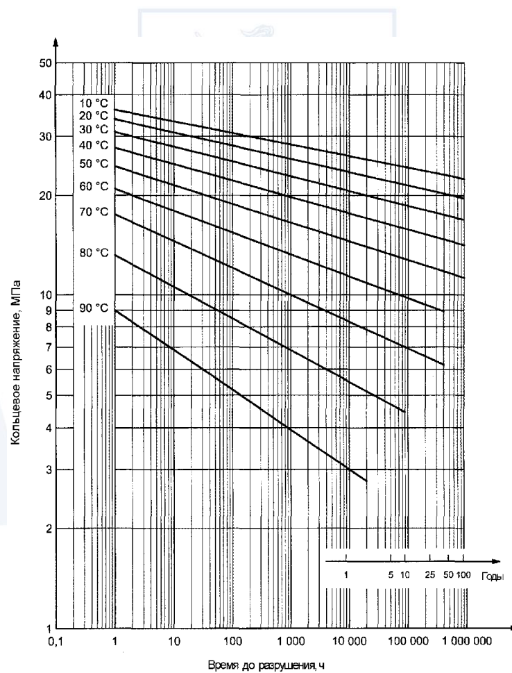
Рисунок В.7. Эталонные графики длительной прочности материала труб PVC-C тип I
