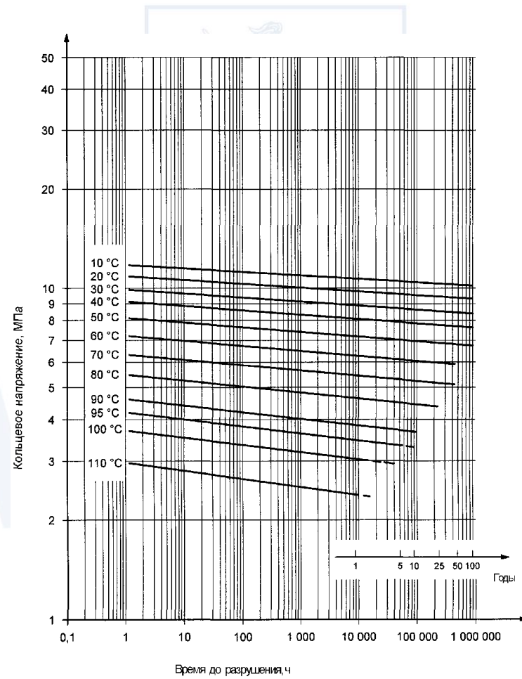
Рисунок В.11. Эталонные графики длительной прочности PE-RT тип I
